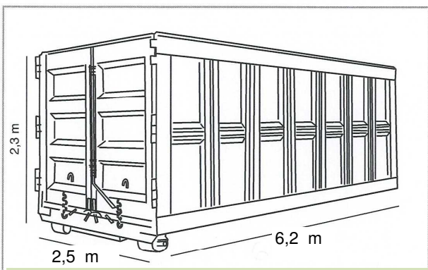
Container da mc 28 per il deposito di rifiuti misti non pericolosi con apertura posteriore a libro.
