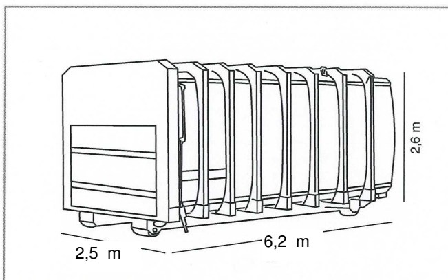
Container da mc 26 predisposto per essere accoppiato alla pressa stazionaria.
