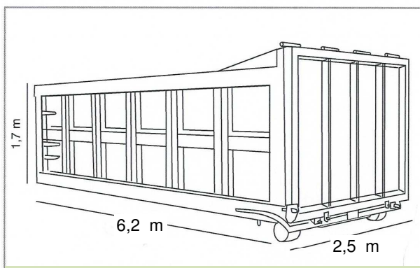
Container da mc 18 a tenuta, a cielo aperto, idoneo al deposito di fanghi. Apertura posteriore basculante.
