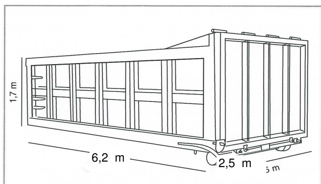
Container rinforzati con misure standard (18 e 28 mc), omologati presso la motorizzazione civile. Idoneo al trasporto di rifiuti pericolosi in regime ADR:
