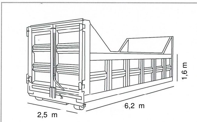
Container da mc 12, a cielo aperto, ideale per il deposito di macerie e materiali ad alto peso specifico.
