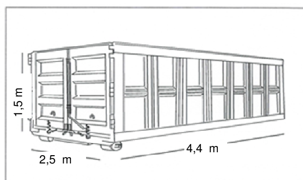
Container da 10 mc a cielo aperto per il deposito di rifiuti, macerie con apertura posteriore a libro.
