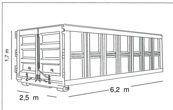
Container da mc 18 per il deposito di rifiuti misti non pericolosi con apertura posteriore a libro.
