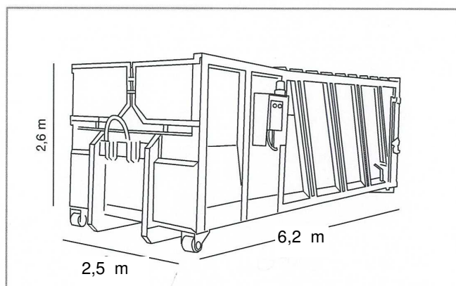
Press Container: container da mc22 predisposto con impianto di compattazione azionato elettricamente per la riduzione volumetrica dei rifiuti.
