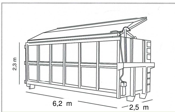
Container da mc 28 coperto per il deposito di rifiuti misti non pericolosi.
