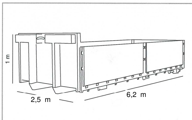
Pianale scarrabile con sponde ribaltabili idoneo per il caricamento di materiali su bancali e in fusti.
